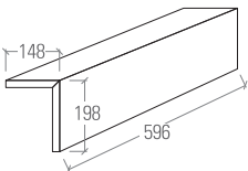
Cordolo "L" 60x20x15
